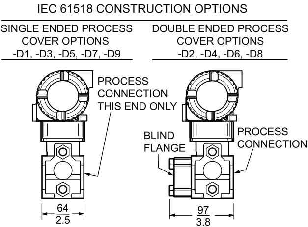
Figure 28 - Biplanar AP/GP Transmitters with Options -D1, -D2, -D3, -D4, -D5, -D6, -D7, -D8, and -D9
